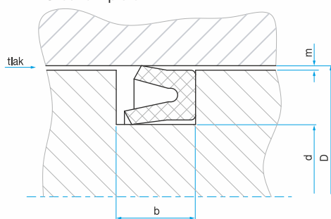
Utěsnění pístu
