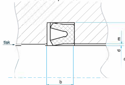
Utěsnění pístnice
