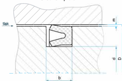
Utěsnění pístu
