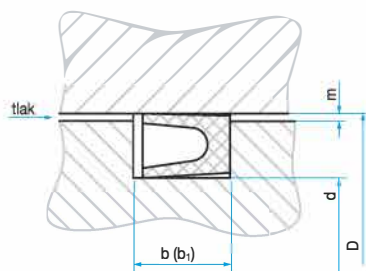
Utěsnění pístu
