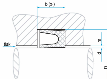
Utěsnění pístnice
